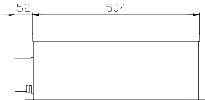
Spodní pohled
