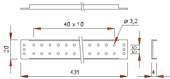
Nosník II. - Fe tl. 1 mm
