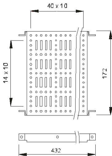
Subpanel U3 - Fe tl. 1 mm
