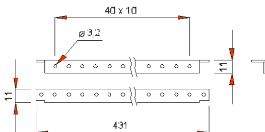
Subpanel U4 - Fe tl. 1 mm
