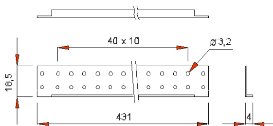
Nosník III. - Fe tl. 1 mm
