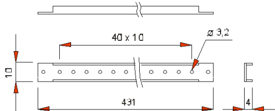
Nosník II. - Fe tl. 1 mm
